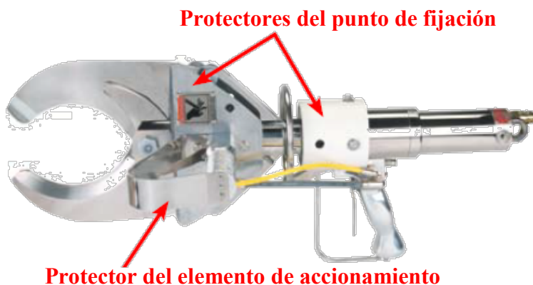
Modelo 30CL-2 Pistola de agarre
